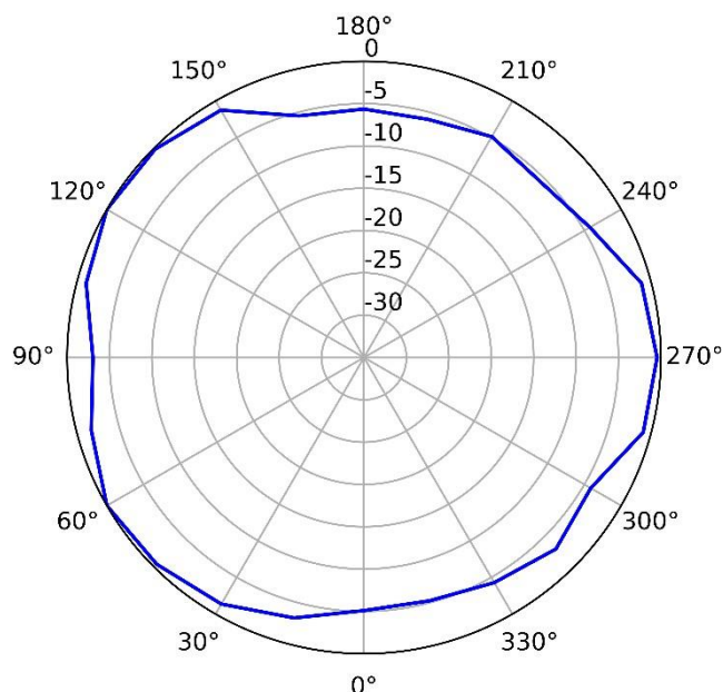
2.4 GHz (vertical)
