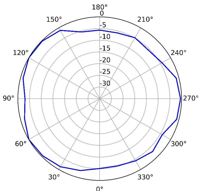
2.4 GHz (vertical)
