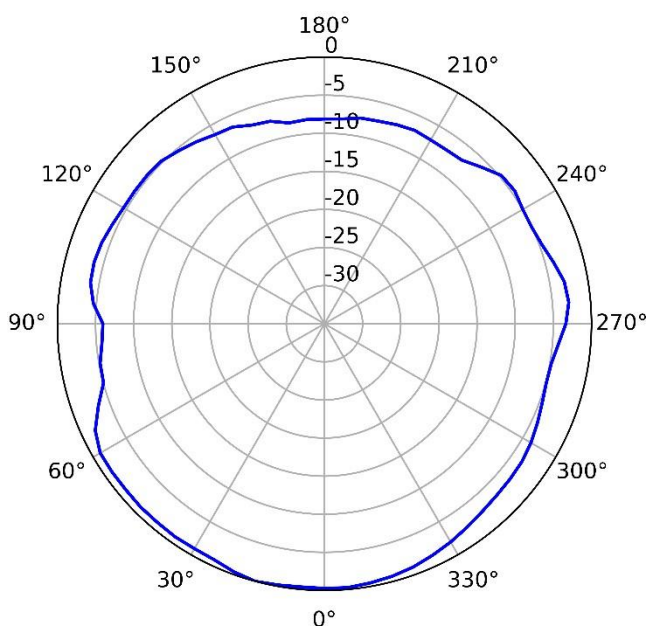
2.4 GHz (horizontal)
